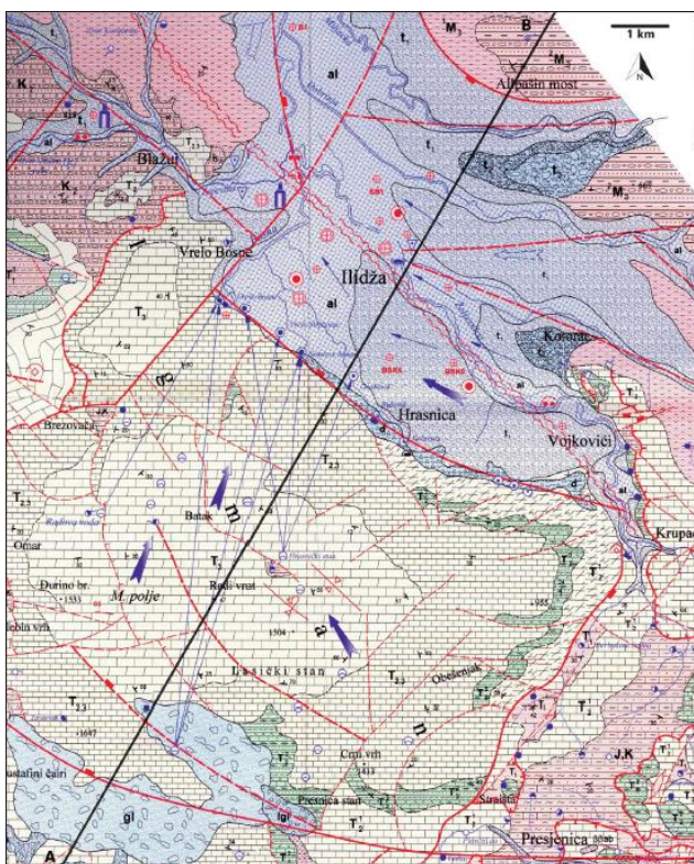
Slika 5. Hidrogeološka karta područja Ilidže
